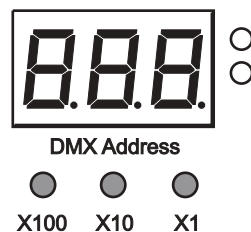
Touches d'adressage du Mania SCX500
